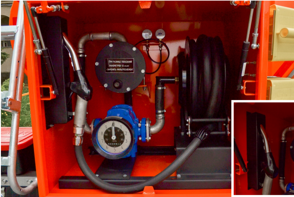
Раздаточный пистолет А-50М
